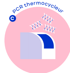
C L'analyse par PCR consiste en une succession de réactions qui permettent la multiplication d'un fragment d'ADN...
