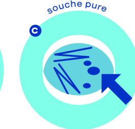
Les colonies sont étalées sur un nouveau milieu de culture afin d'obtenir des souches pures C . Les souches pures peuvent être ensuite analysées par PCR, voir méthode suivante 3 .
